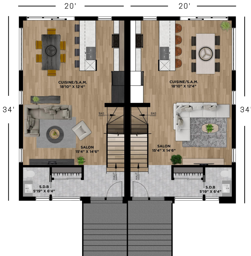
REZ-DE-CHAUSSÉE
